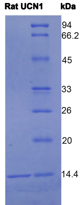
15% SDS-PAGE
