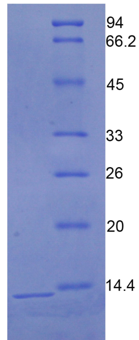
15% SDS-PAGE
