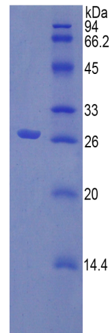
15% SDS-PAGE
