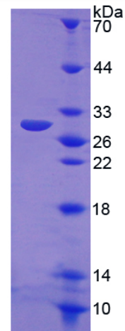
15% SDS-PAGE
